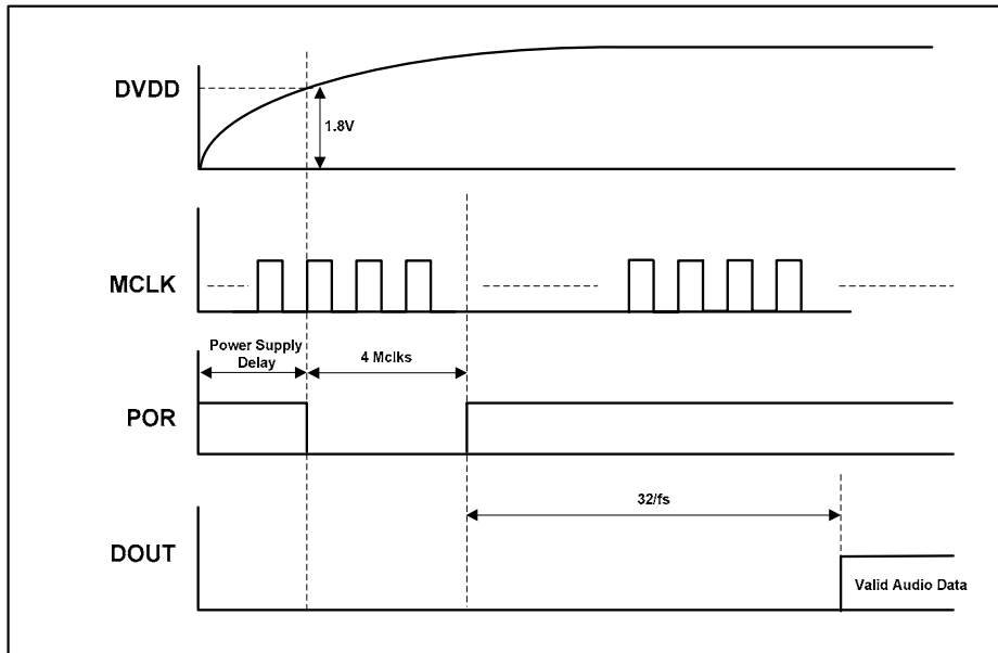
Figure 7 POR Timing
