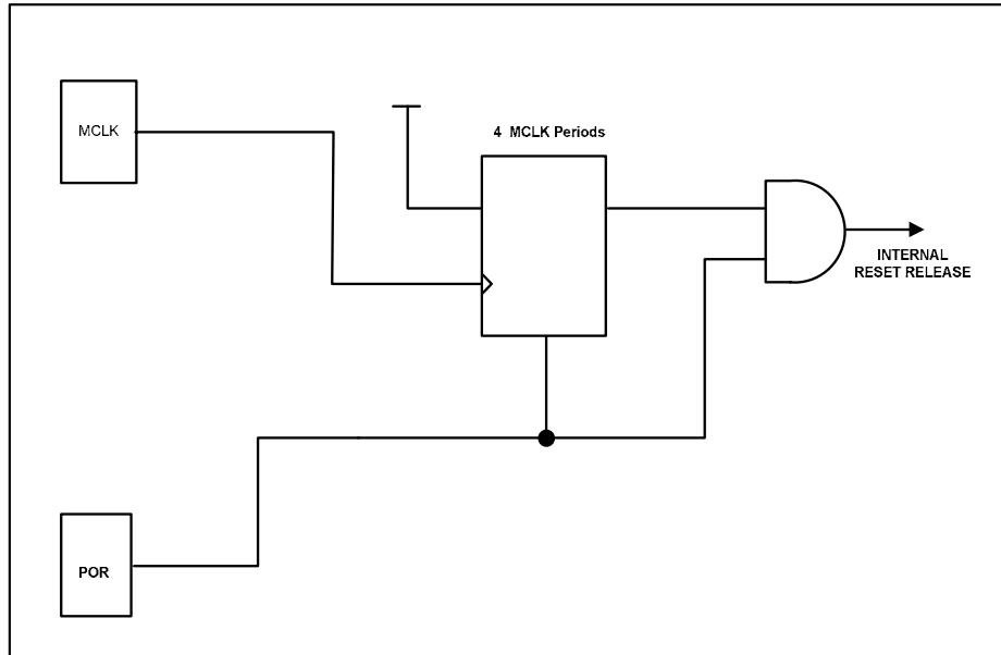
Figure 6 POR Circuit
